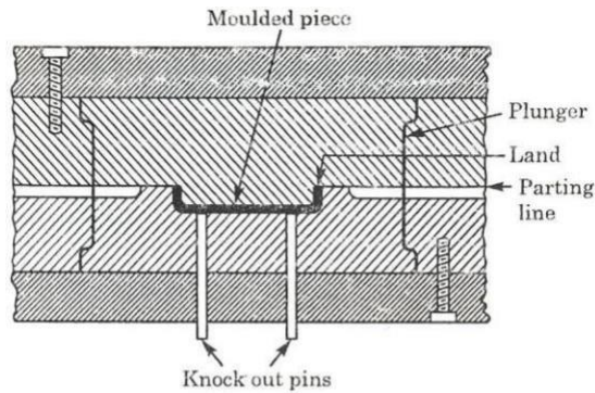
Fig. 4.1. Flash type.
